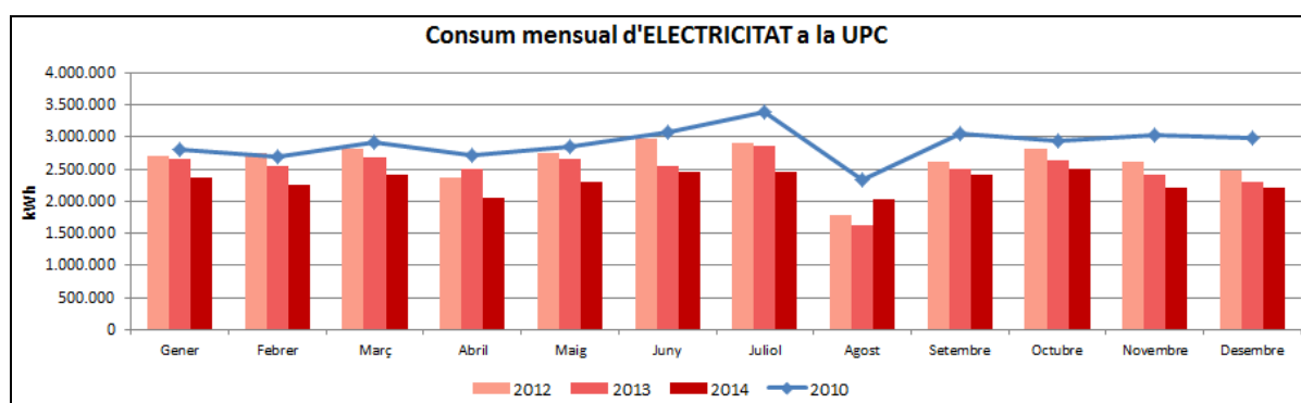
Fig.13. Evolució del consum elèctric de la UPC de forma mensual.
